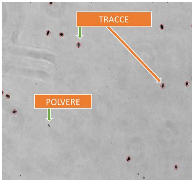
Figura 2. Immagine al microscopio delle tracce di particelle alfa emesse dal radon sulla superficie del CR-39 dopo trattamento chimico.
